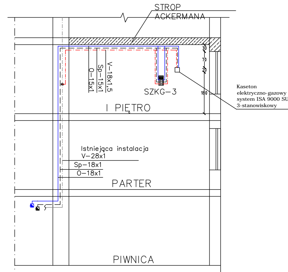
PRZEKRÓJ A-A
